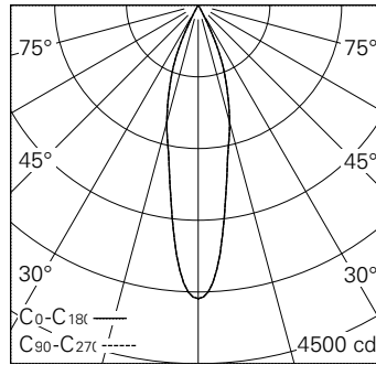
LED 2700 K 11 W 903 lm-h 24° / CIE Flux 100 100 100 100 100 / A80 nach DIN 5040
