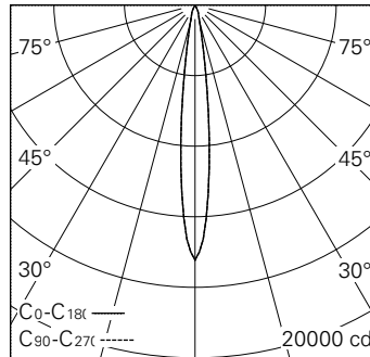
LED 4000 K 11 W 1129 lm-h 12.6° / CIE Flux 100 100 100 100 100 / A80 nach DIN 5...
