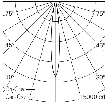
LED 2700 K 11 W 872 lm-h 12.6° / CIE Flux 100 100 100 100 100 / A80 nach DIN 5040
