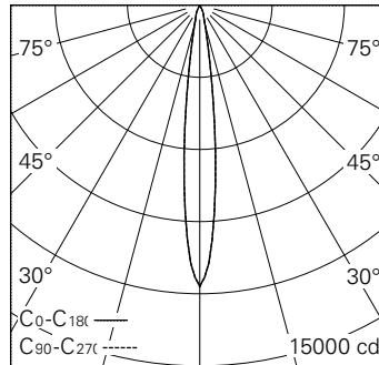
LED 3000 K 11 W 913 lm-h 12.6° / CIE Flux 100 100 100 100 100 / A80 nach DIN 5040
