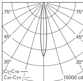
LED 3000 K 11 W 797 lm-h 12.6° / CIE Flux 100 100 100 100 100 / A80 nach DIN 5040
