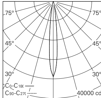
LED 4000 K 20 W 1968 lm-h 11.6° / CIE Flux 100 100 100 100 100 / A80 nach DIN 5...
