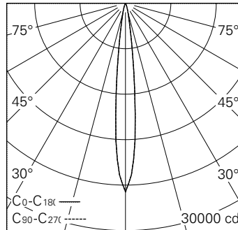
LED 3000 K 20 W 1574 lm-h 11.6° / CIE Flux 100 100 100 100 100 / A80 nach DIN 5...
