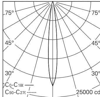
LED 3000 K 20 W 1394 lm-h 11.6° / CIE Flux 100 100 100 100 100 / A80 nach DIN 5...
