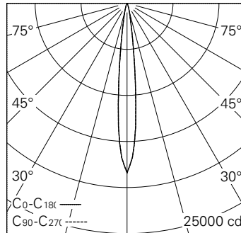
LED 3000 K 14 W 1164 lm-h 11.6° / CIE Flux 100 100 100 100 100 / A80 nach DIN 5...
