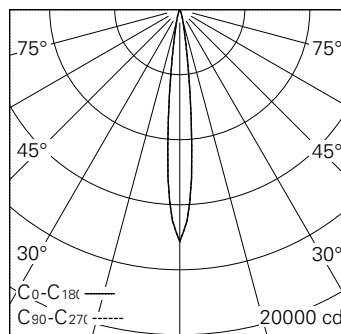
LED 3000 K 11 W 902 lm-h 11.6° / CIE Flux 100 100 100 100 / A80 nach DIN 5040
