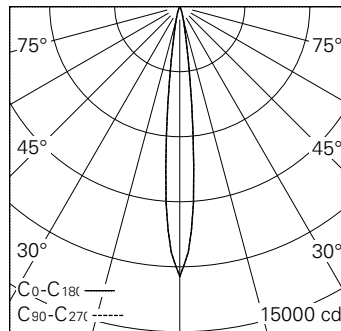
LED 3000 K 11 W 787 lm-h 11.6° / CIE Flux 100 100 100 100 100 / A80 nach DIN 5040
