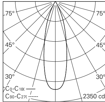
LED 4000 K 11 W 620 lm-h 30° / CIE Flux 99 100 100 100 100 / A80 nach DIN 5040
