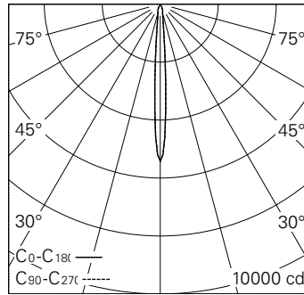
LED 2700 K 4,6 W 303 lm-h 8.0° / CIE Flux 100 100 100 100 100 / A80 nach DIN 5040
