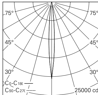
LED 4000 K 11 W 753 lm-h 8.2° / CIE Flux 100 100 100 100 100 / A80 nach DIN 5040
