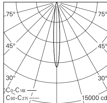
LED 4000 K 9,3 W 689 lm-h 11.0° / CIE Flux 99 100 100 100 / A80 nach DIN 5040
