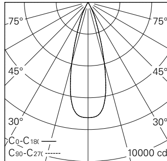
LED 3000 K 27 W 2154 lm-h 32° / CIE Flux 100 100 100 100 100 / A80 nach DIN 5040
