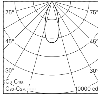
LED 2700 K 20 W 1995 lm-h 38° / CIE Flux 98 100 100 100 100 / A80 nach DIN 5040
