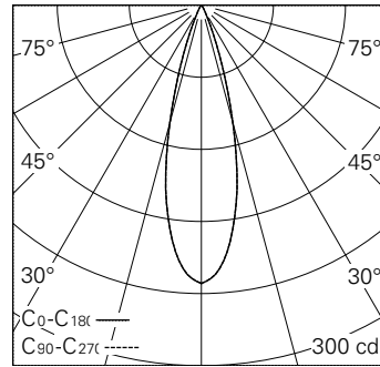
LED 2700 K 2,6 W 56 lm-h 28° / CIE Flux 99 100 100 100 100 / A80 nach DIN 5040
