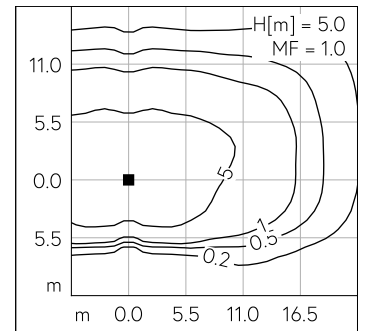
LED 4000 K 26.1 W 3688 lm-h H = 5 m / CIE Flux 38 75 96 100 100 / A30 nach DIN ...
