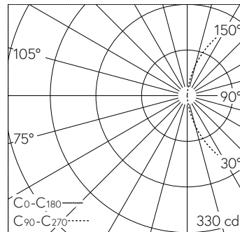
LED 3000 K 14 W 1146 lm-h / CIE Flux 13 37 66 50 100 / C11 nach DIN 5040
