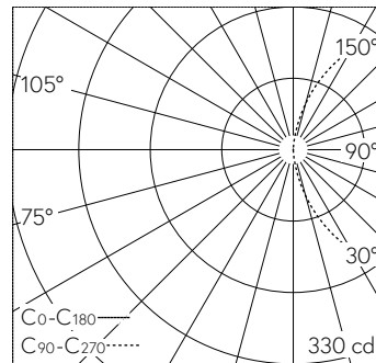
LED 3000 K 14 W 1130 lm-h / CIE Flux 13 37 66 50 100 / C11 nach DIN 5040
