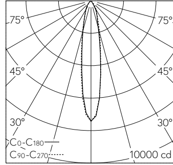
LED 4000 K 19 W 1725 lm-h 71118M / CIE Flux 94 99 100 100 100 / A80 nach DIN 5...
