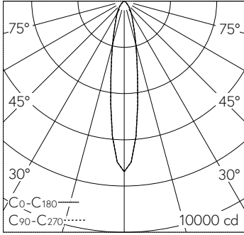
LED 4000 K 19 W 1937 lm-h 18.4° / CIE Flux 89 99 100 100 100 / A80 nach DIN 5040
