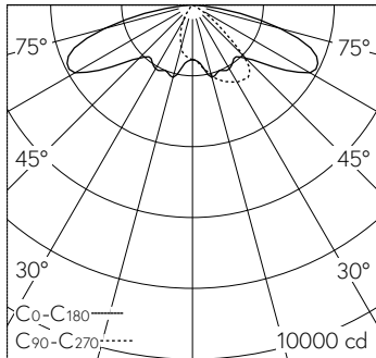
LED 3000 K 69 W 9163 lm-h H = 8 m / CIE Flux 34 66 93 100 100 / A20 nach DIN 5...
