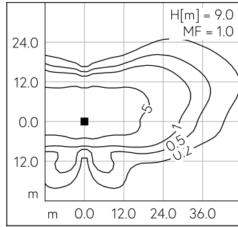
LED 3000 K 69 W 9163 lm-h H = 9 m / CIE Flux 34 66 93 100 100 / A20 nach DIN 5...
