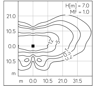
LED 3000 K 69 W 9163 lm-h H = 7 m / CIE Flux 34 66 93 100 100 / A20 nach DIN 5...
