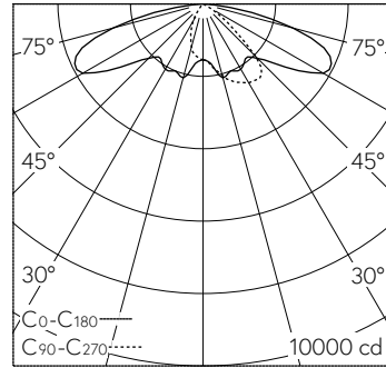
LED 3000 K 69 W 9163 lm-h H = 7 m / CIE Flux 34 66 93 100 100 / A20 nach DIN 5...
