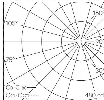
LED 3000 K 25 W 1651 lm-h / CIE Flux 13 37 66 50 100 / C11 nach DIN 5040
