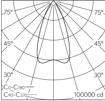
LED 4000 K 326 W 42233 lm-h 48° / CIE Flux 99 100 100 100 100 / A80 nach DIN 5...
