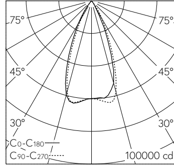
LED 4000 K 326 W 35130 lm-h 71101M / CIE Flux 99 100 100 100 100 / A80 nach DI...
