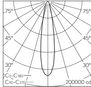
LED 4000 K 326 W 41334 lm-h 22° / CIE Flux 98 100 100 100 100 / A80 nach DIN 5... LED 4000 K 326 W 33056 lm-h 71101M / CIE Flux 98 100 100 100 100 / A80 nach D...
