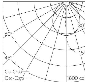
LED 3000 K 20 W 2523 lm-h / CIE Flux 41 77 96 100 100 / A30 nach DIN 5040
