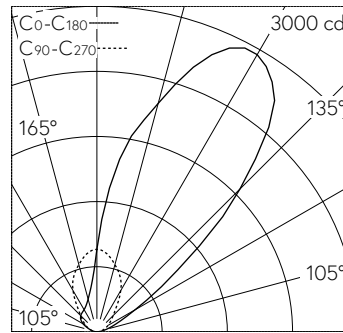
LED 4000 K 35.3 W 2847 lm-h / CIE Flux 0 0 0 100 / E84 nach DIN 5040
