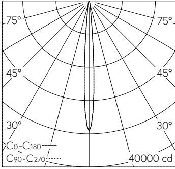
LED 4000 K 20.9 W 1244 lm-h 8.4° / CIE Flux 99 100 100 100 100 / A80 nach DIN 5...
