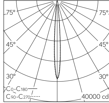
LED 4000 K 20.9 W 1220 lm-h 71118M / CIE Flux 99 100 100 100 100 / A80 nach DI...
