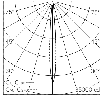
LED 3000 K 20.3 W 1201 lm-h 71118M / CIE Flux 99 100 100 100 100 / A80 nach DI...
