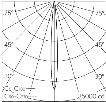
LED 3000 K 20.3 W 1225 lm-h 8.4° / CIE Flux 99 100 100 100 100 / A80 nach DIN 5...
