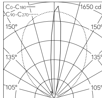
LED RGBW 0 K 17 W 608 lm-h / CIE Flux 0 0 0 100 / E84 nach DIN 5040
