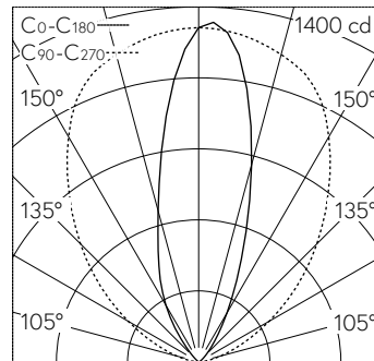
LED RGBW 0 K 28 W 1279 lm-h / CIE Flux 0 0 17 0 100 / E84 nach DIN 5040
