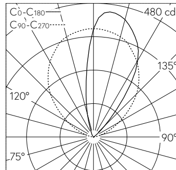
LED RGBW 0 K 17 W 485 lm-h / CIE Flux 0 0 20 0 100 / E84 nach DIN 5040
