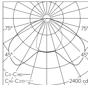
LED 4000 K 86.2 W 10408 lm-h / CIE Flux 41 79 97 100 100 / A30 nach DIN 5040
