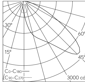
LED 4000 K 22 W 2661 lm-h / CIE Flux 39 81 97 100 100 / A30 nach DIN 5040
