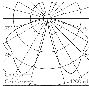
LED 3000 K 43.5 W 2641 lm-h / CIE Flux 36 68 93 99 100 / A30 nach DIN 5040
