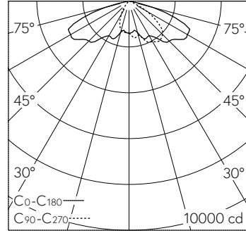
LED 4000 K 53 W 7770 lm-h H = 8 m / CIE Flux 33 72 98 100 100 / A20 nach DIN 5...
