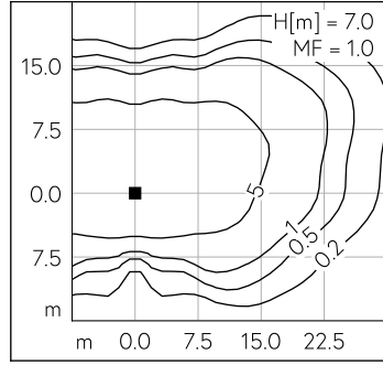
LED 4000 K 53 W 7770 lm-h H = 7 m / CIE Flux 33 72 98 100 100 / A20 nach DIN 5...
