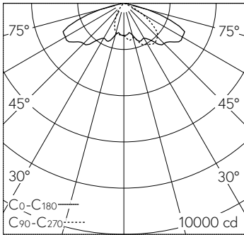
LED 4000 K 53 W 7770 lm-h H = 9 m / CIE Flux 33 72 98 100 100 / A20 nach DIN 5...
