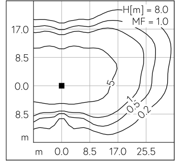
LED 4000 K 53 W 7770 lm-h H = 8 m / CIE Flux 33 72 98 100 100 / A20 nach DIN 5...
