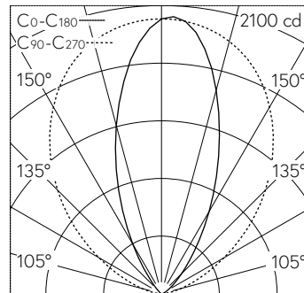
LED 3000 K 28 W 2350 lm-h / CIE Flux 0 0 3 0 100 / E84 nach DIN 5040
