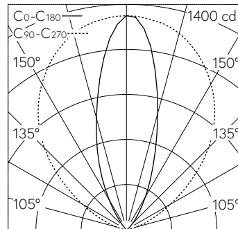
LED 3000 K 15.5 W 1251 lm-h / E84 nach DIN 5040
