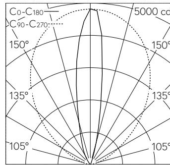
LED 3000 K 28 W 2743 lm-h / CIE Flux 0 14 14 0 100 / E84 nach DIN 5040
