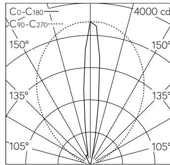
LED 4000 K 15.5 W 1379 lm-h / CIE Flux 0 0 4 0 100 / E84 nach DIN 5040
