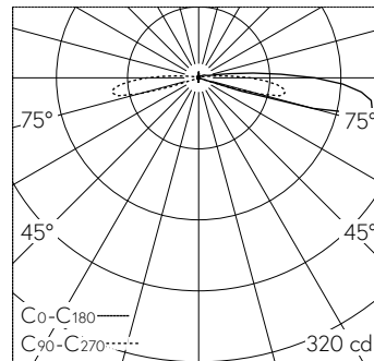
LED 2700 K 7 W 176 lm-h / CIE Flux 1 2 16 74 100 / B11 nach DIN 5040
