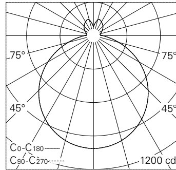
LED 4000 K 35 W 3700 lm-h / CIE Flux 45 75 92 84 100 / B43 nach DIN 5040
