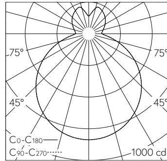
LED 4000 K 35 W 3660 lm-h / CIE Flux 43 73 91 74 100 / B32 nach DIN 5040
