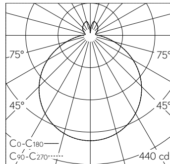
LED 3000 K 13.3 W 1285 lm-h / CIE Flux 45 75 92 86 100 / B42 nach DIN 5040
