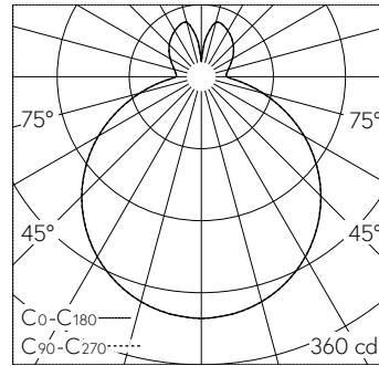
LED 3000 K 13.3 W 1256 lm-h / CIE Flux 43 73 91 77 100 / B32 nach DIN 5040
