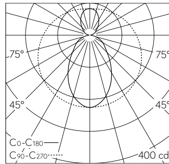
LED 3000 K 32.6 W 1125 lm-h / CIE Flux 39 65 84 64 100 / B32 nach DIN 5040
