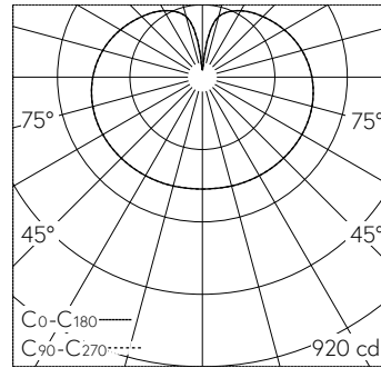
LED 3000 K 39.5 W 4098 lm-h / CIE Flux 25 50 75 55 100 / C12 nach DIN 5040
