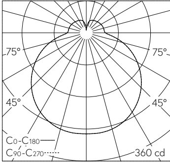
LED 4000 K 25 W 1531 lm-h / CIE Flux 39 68 88 78 100 / B32 nach DIN 5040
