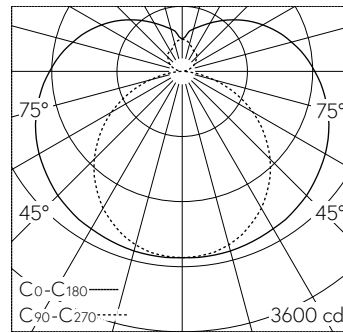
LED 3000 K 147 W 16223 lm-h / CIE Flux 34 61 82 69 100 / B21 nach DIN 5040
